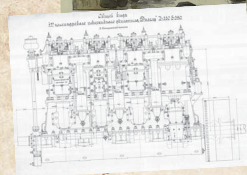
Общий вид 4-цилиндрового реверсивного двигателя. Завод «Людвиг Нобель». 1909 г. ЦГАНТД СПб
